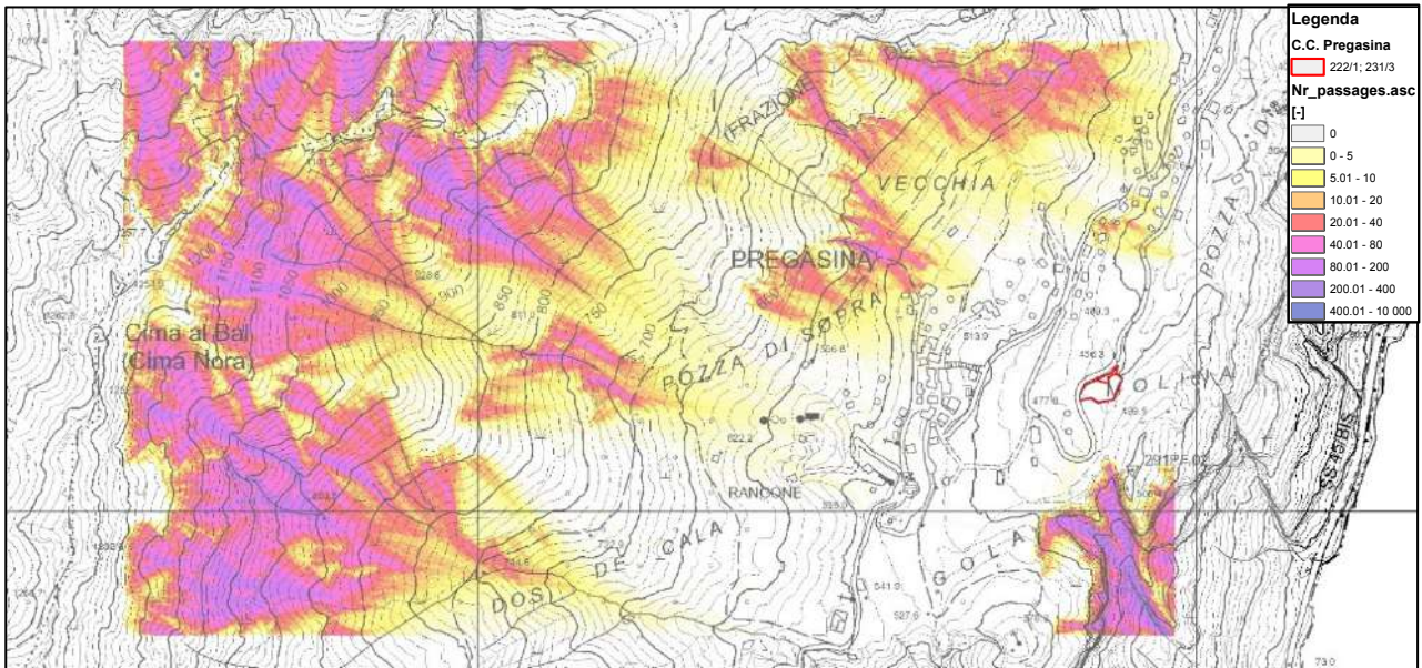
Figura Errore. Nel documento non esiste testo dello stile specificato..7 - numero di blocchi in transito per singola cella Scenario 2 – blocco sferico
