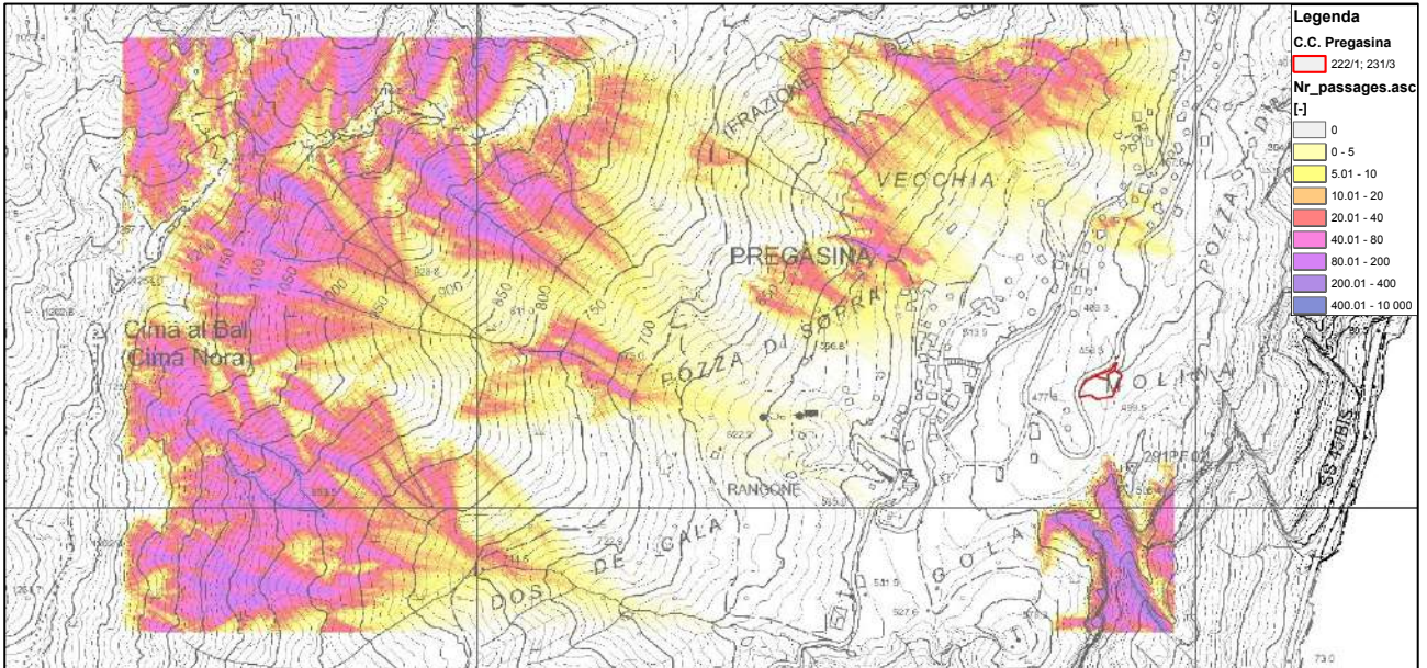
Figura Errore. Nel documento non esiste testo dello stile specificato.3 - numero di blocchi in transito per singola cella Scenario 1 – blocco prismatico
