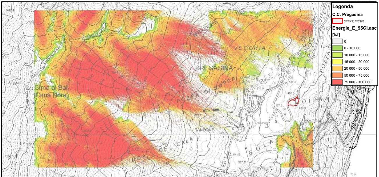
Figura Errore. Nel documento non esiste testo dello stile specificato..5 – massime energie 95%CL delle traiettorie di crollo Scenario 1 – blocco prismatico
