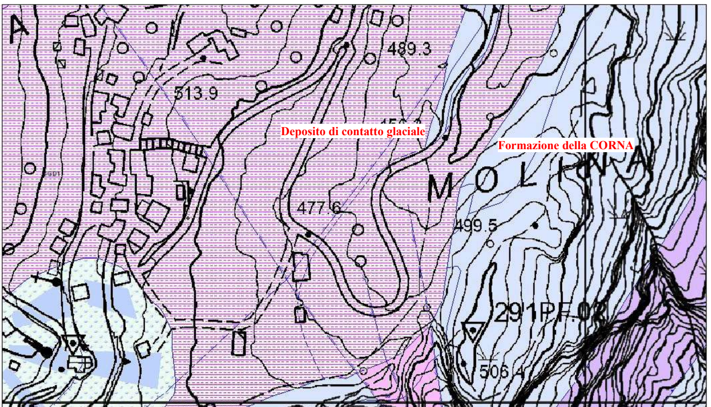
Carta Geologica
